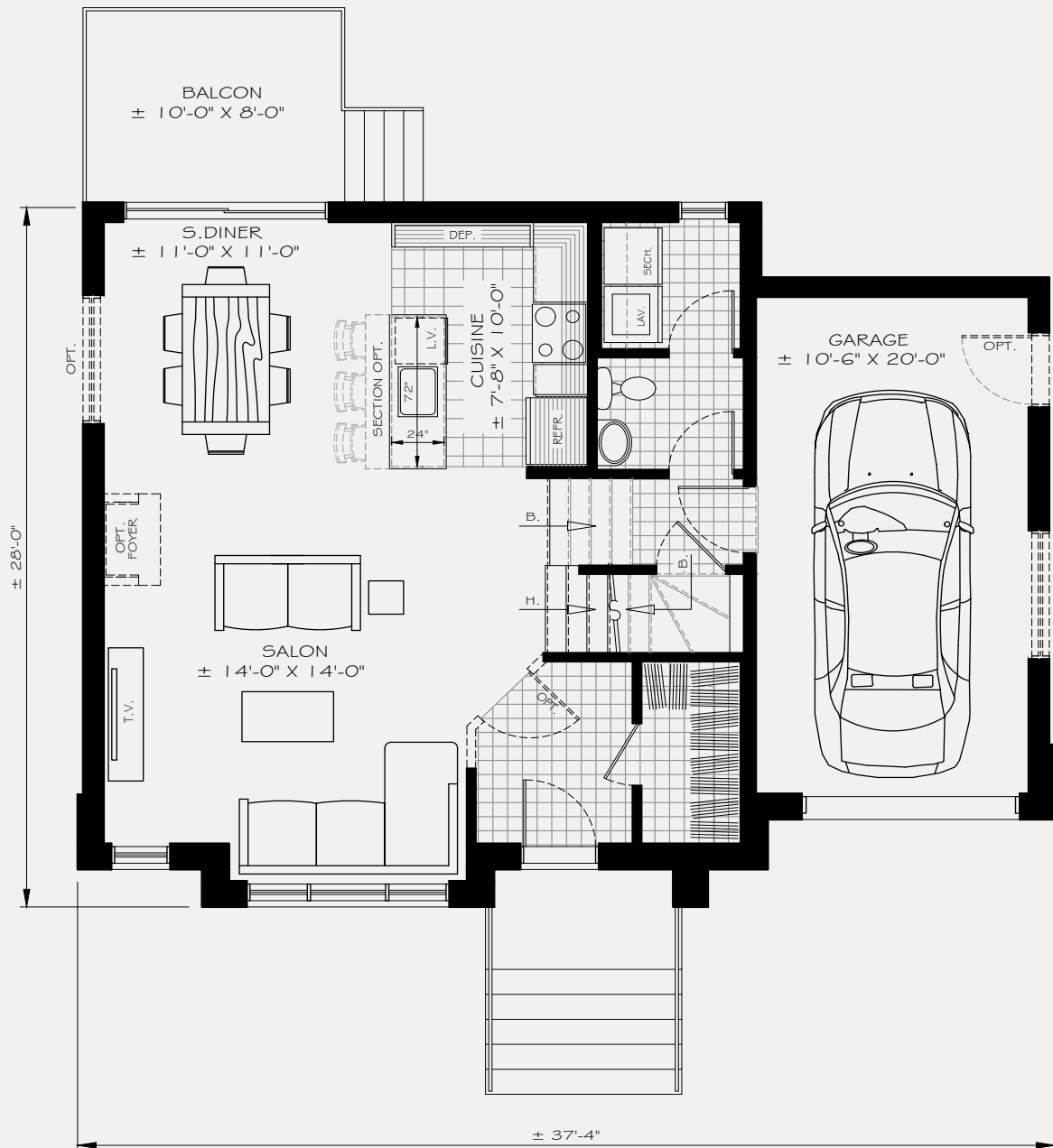
REZ-DE-CHAUSSÉE 692 PI.CA
